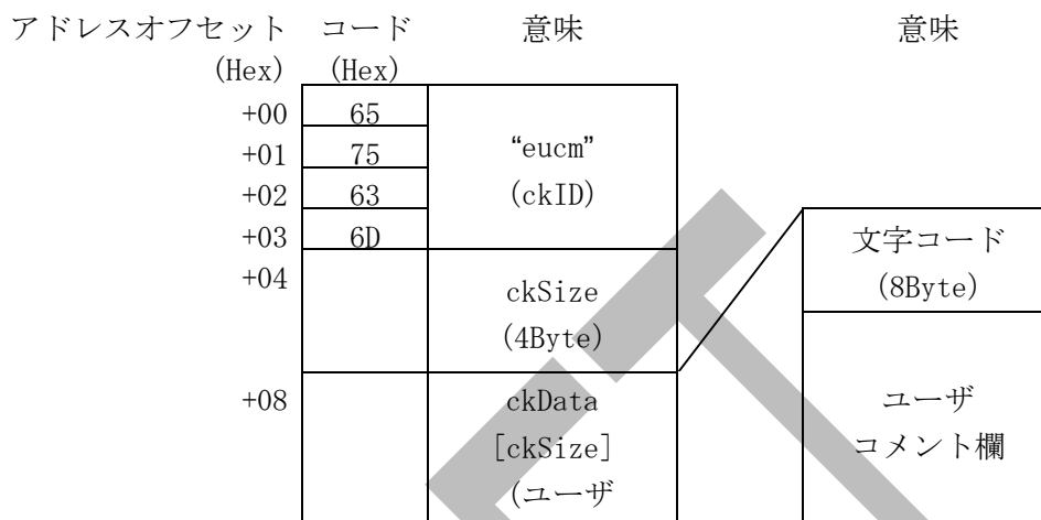
図 56 ユーザコメントチャンクの構造
