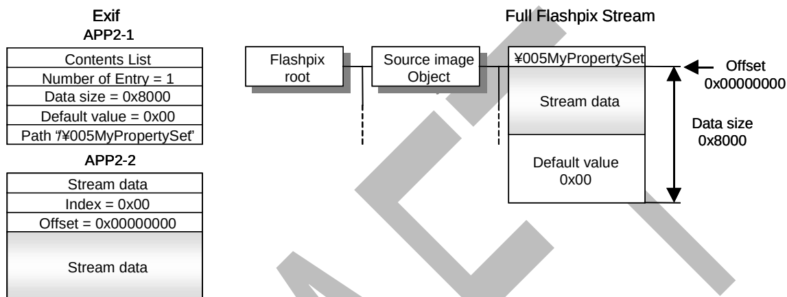
図 63 Flashpix 拡張データ変換例 (1)
