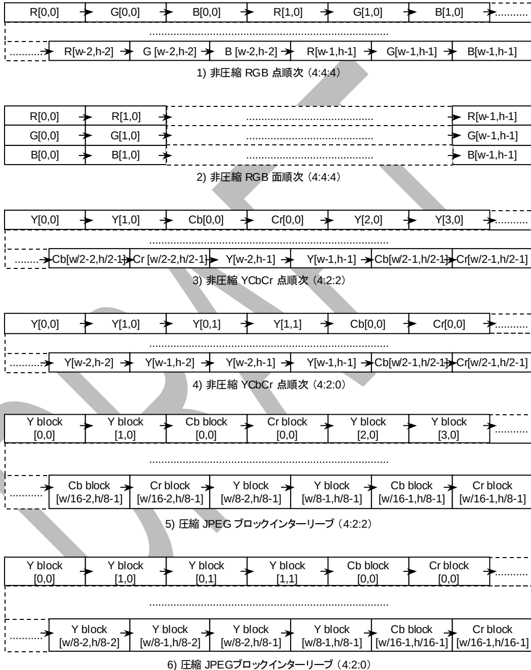
図 5 データの並び
