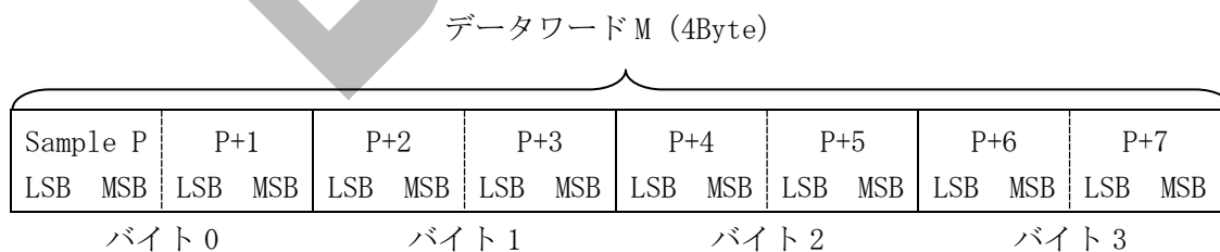
図 53 IMA-ADPCM 音声データのデータワード M
