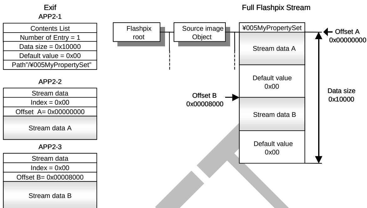
図 64 Flashpix 拡張データ変換例 (2)
