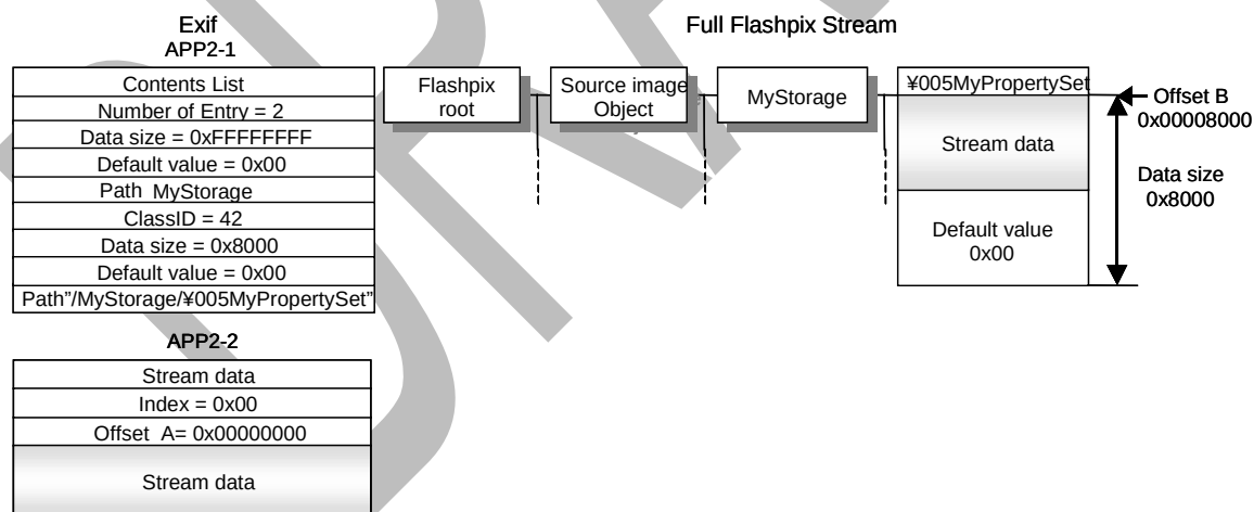
図 65 Flashpix 拡張データ変換例 (3)
