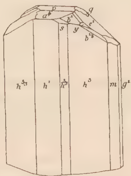
Fig. 1 et 2. Hambergite d'Imalo.
