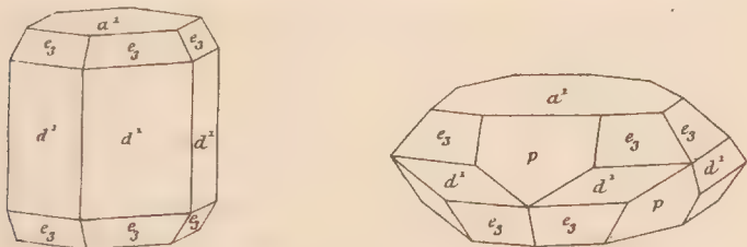
Fig. 1 et 2. Corindon d'Ambatovy.
