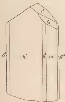
Fig. 1 et 2. Hambergite d'Imalo.
