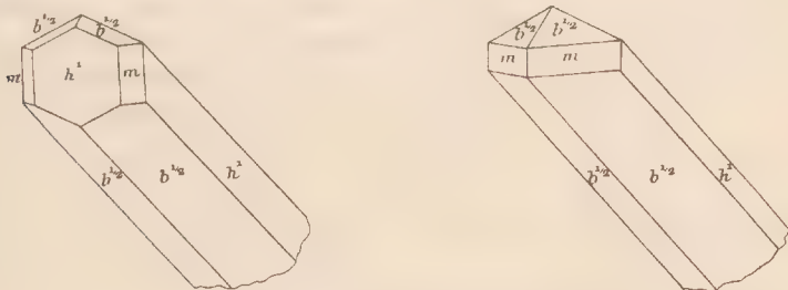
Fig. 1 et 2. Strüvérite d'Ampangabé (Type II).
