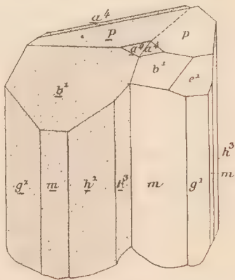
Fig. 3. Macie suivant m (110) de la hambergite d'Imalo.
