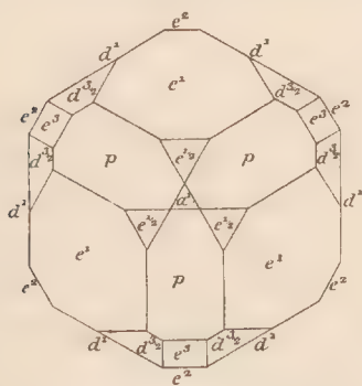
Fig. 6. Tourmaline noire d'Ambatomainity (projection sur la base).
