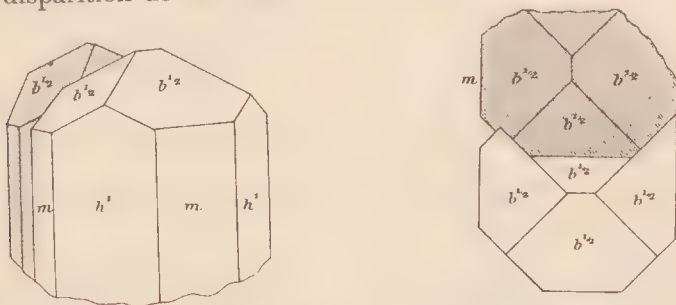
Fig. 3 et 4. Groupement à axes parallèles de cristaux du type I de la strüvérite d'Ampangabé (fig. 4, projection sur la base).
