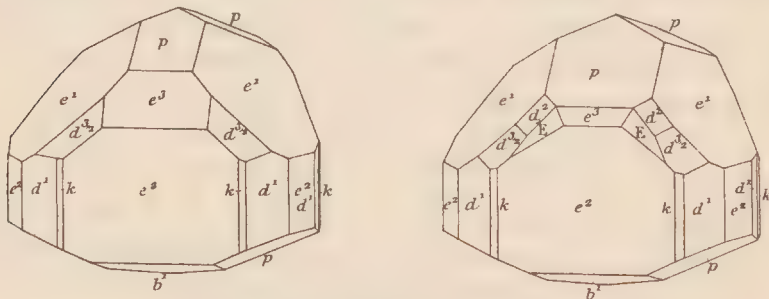
Fig. 1 et 2. — Tourmaline noire d'Ambatomainity.
