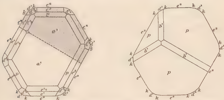
Fig. 4 et 5. — Projection sur la base des deux extrémités d'une macle de tourmaline noire d'Ambatomainity.
