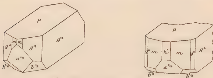
Fig. 1 et 2. — Orthose ferrière d'Itrongahy.
